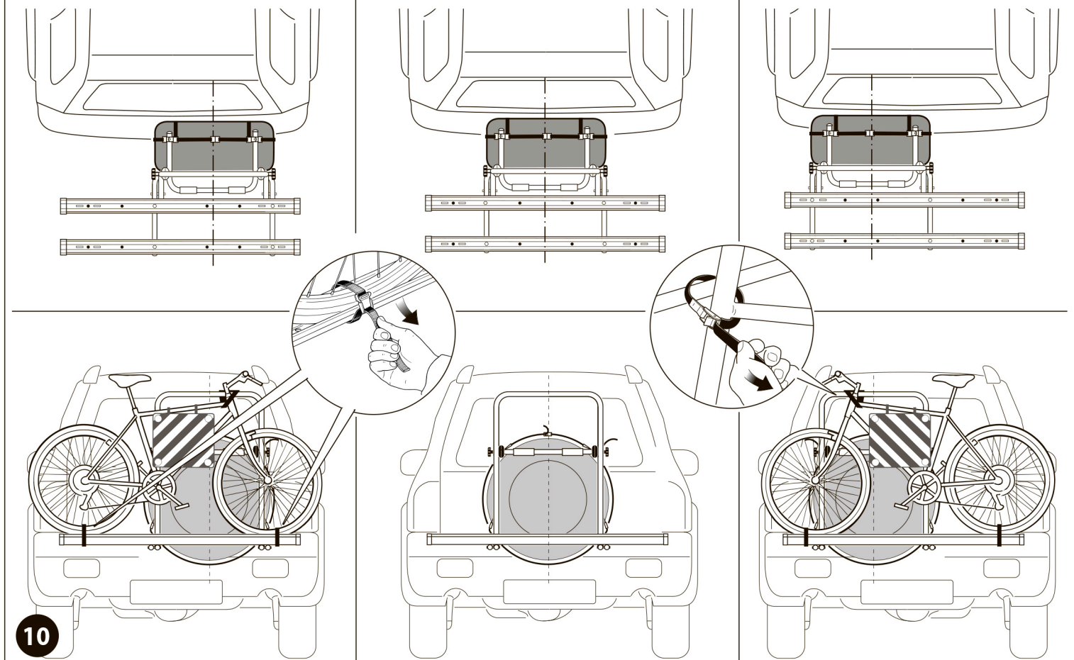
ЗАПАСНОЕ КОЛЕСО СПРАВА SPARE WHEEL RIGHT RUEDA A LA DERECHA
