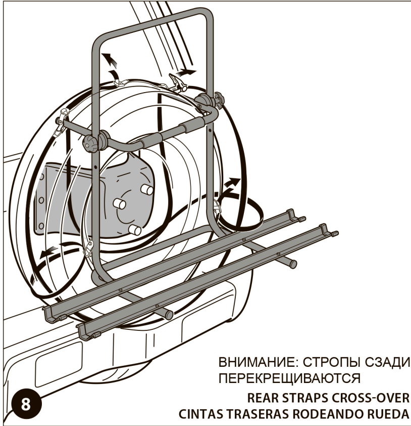
ЗАПАСНОЕ КОЛЕСО СПРАВА SPARE WHEEL RIGHT RUEDA A LA DERECHA
